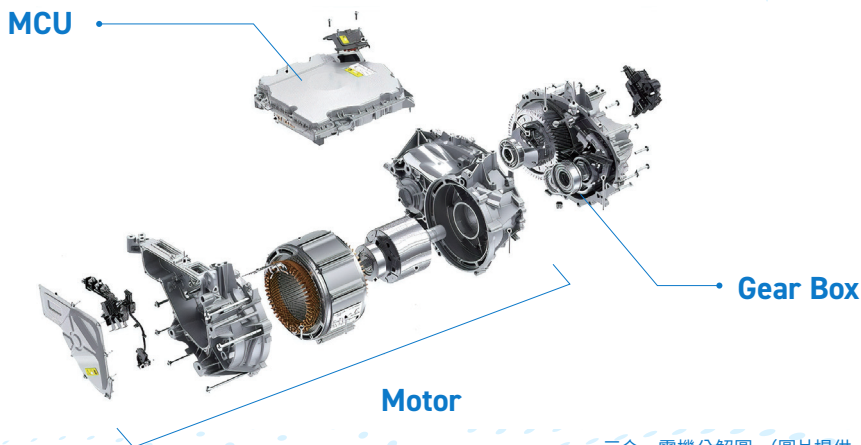
三合一電機分解圖。(圖片提供：鴻華)
