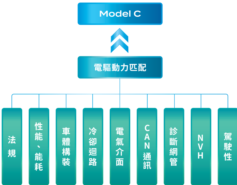
電驅動力匹配架構圖。(圖片提供：鴻華)
