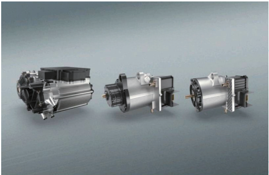
信通旗下的微型移動解決方案電機產品，以在地製造兼顧可靠性與成本效益，為二輪與三輪車市場提供高效率動力支援。(圖片提供：信通)
