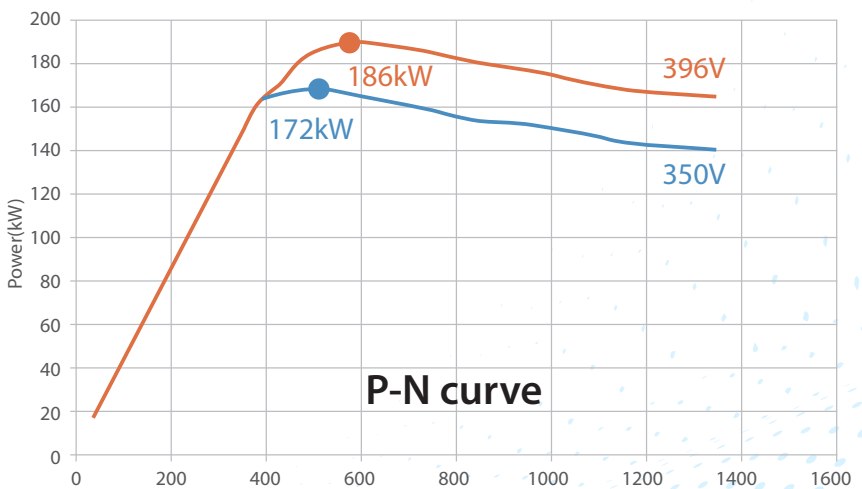
電機峰值功率曲線圖。(圖片提供：鴻華)
